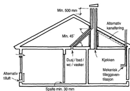
Figur 3 Prinsipp tegning bolig naturlig ventilasjon
