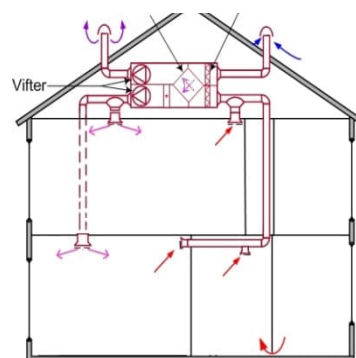
Figur 5 Prinsipp tegning bolig mekanisk ventilasjon
