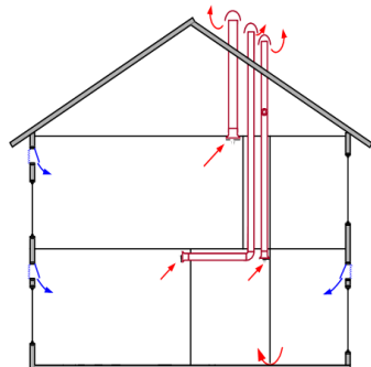
Figur 2 Naturlig avtrekksventilasjon
