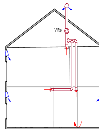
Figur 4 Mekanisk ventilasjon
