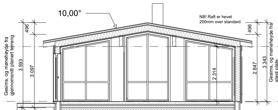
Snitt A-A
