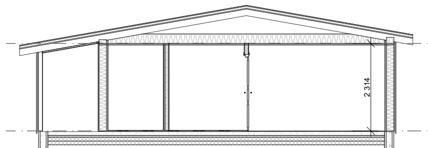
Snitt B-B
