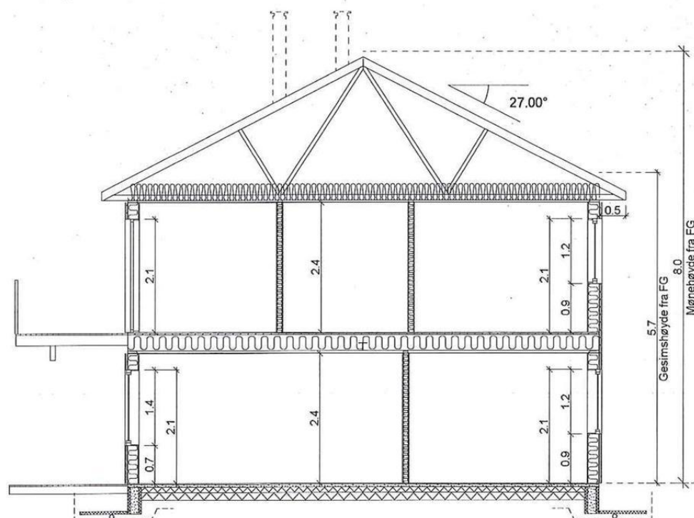
SNITT A-A
