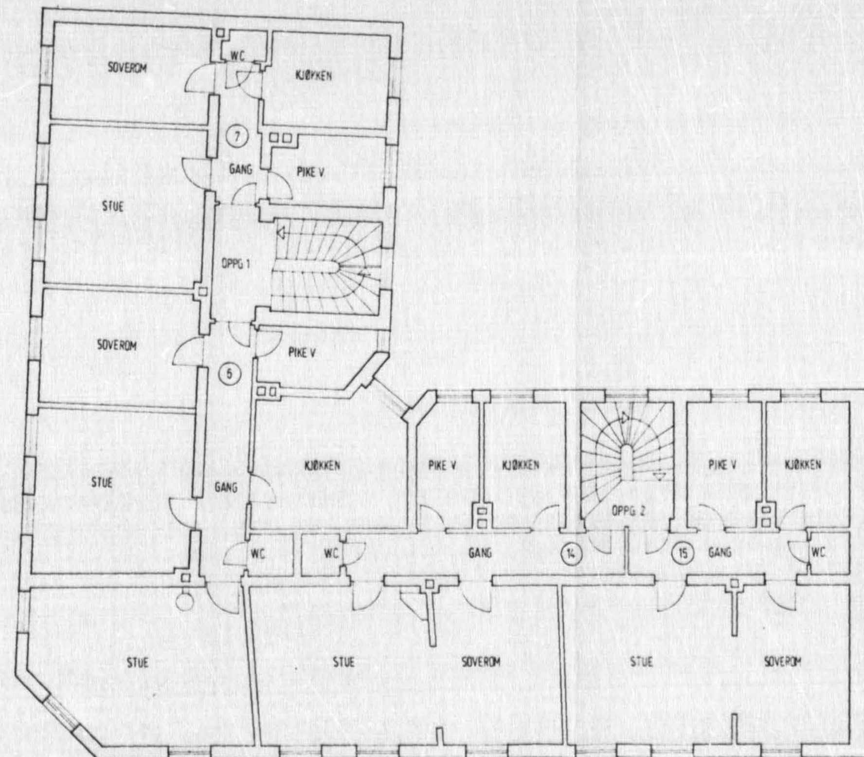
4. ETASJE EKST. PLAN
