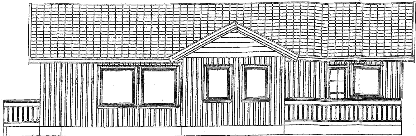
FASADE SØR
