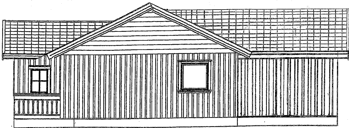
FASADE ØST
